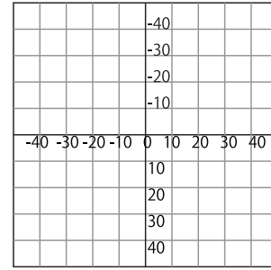
AxisPlane.png (200 × 200px)
